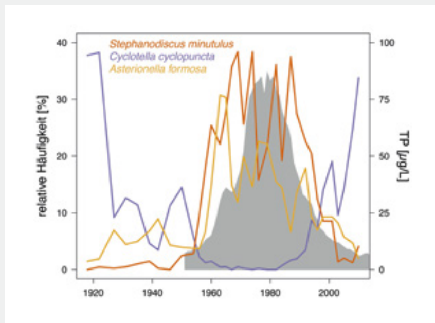
Fig. 2 Entwicklung der relativen Häufigkeit von drei Diatomeenarten ( Stephanodiscus minutulus , Asterionella formosa und Cyclotella cyclopuncta ) und der Gesamtposphor-Konzentration (TP, graue Fläche) während der Eutrophierung und Re-Oligotrophierung des Bodensees. Daten aus [7].
