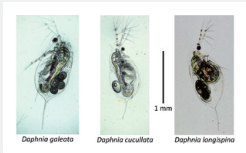
Fig. 4 Die drei Wasserfloharten ( Daphnia ), die im Bodensee vorkommen. (© Piet Spaak, Eawag)
