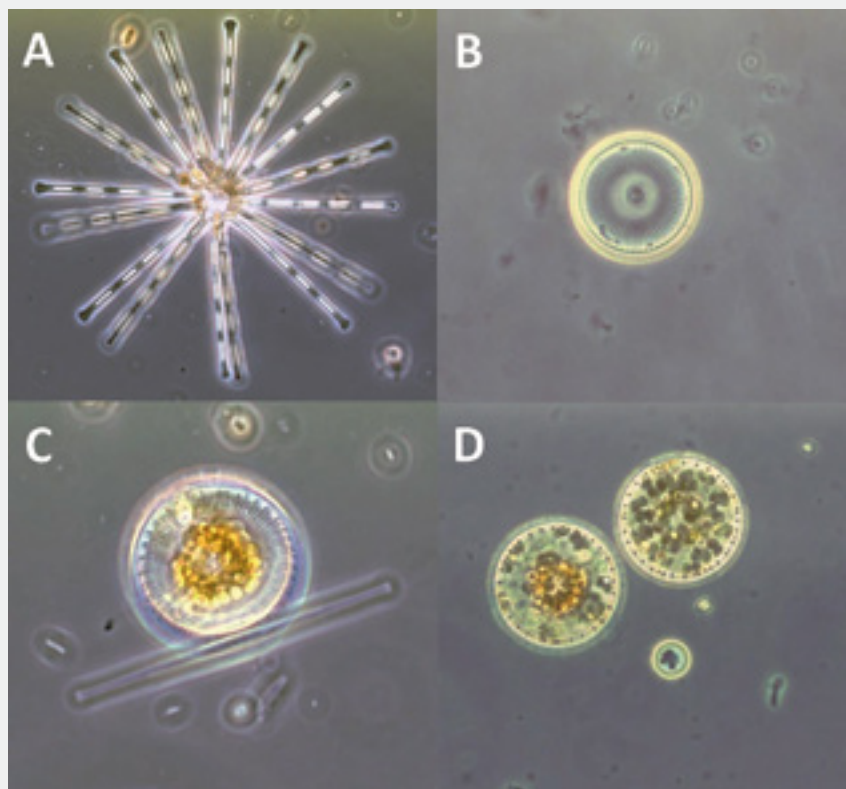
Fig. 3 Kieselalgen aus dem Bodensee: A Asterionella formosa (Koloniedurchmesser 200 µm); B Cyclotella bodanica (Zelldurchmesser ~25 µm); C Stephanodiscus sp. (Zelldurchmesser ~30 µm); D Stephanodiscus neoastraea (Zelldurchmesser ~50 µm).
