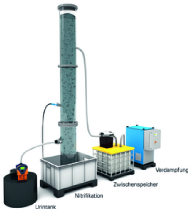
Abb. 2: Die im Projekt «Vuna» entwickelte Technik zur Separierung und Aufbereitung von Urin wird auch bei «Water Hub» eingesetzt. Eine Nitrifikations- und Verdampfungsanlage wandelt den getrennt gesammelten Urin mitsamt seinen Nährstoffen in einen Dünger um. (Bild: Eawag)
