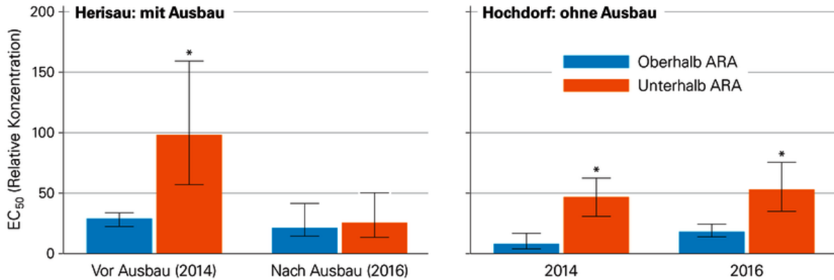
Abb. 3: Die Algen unterhalb der ARA Herisau haben ihre Toleranz gegenüber Mikroverunreinigungen nach dem Ausbau wieder verloren: Sie reagieren schon bei tieferen Effektkonzentrationen (EC 50 ) mit einer verminderten Biomassenproduktion. Dagegen zeigen sich bei der nicht aufgerüsteten ARA Hochdorf zwischen den beiden Messjahren keine Unterschiede. Die EC 50 gibt an, bei welcher Stoffkonzentration 50 Prozent einer Population in einer Lebensfunktion (in diesem Fall bei der Produktion von Biomasse) beeinträchtigt wird. *statistisch signifikante Resultate
