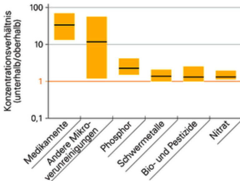
Abb. 2: Verhältnis der unterhalb und oberhalb der Kläranlagen gemessenen Konzentrationen verschiedener Substanzen. Werte >1 bedeuten, dass unterhalb höhere Konzentrationen gemessen wurden als oberhalb. Die schwarzen Linien entsprechen dem Median, die gelben Bereiche einer Abweichung von \pm 25 Prozent.
