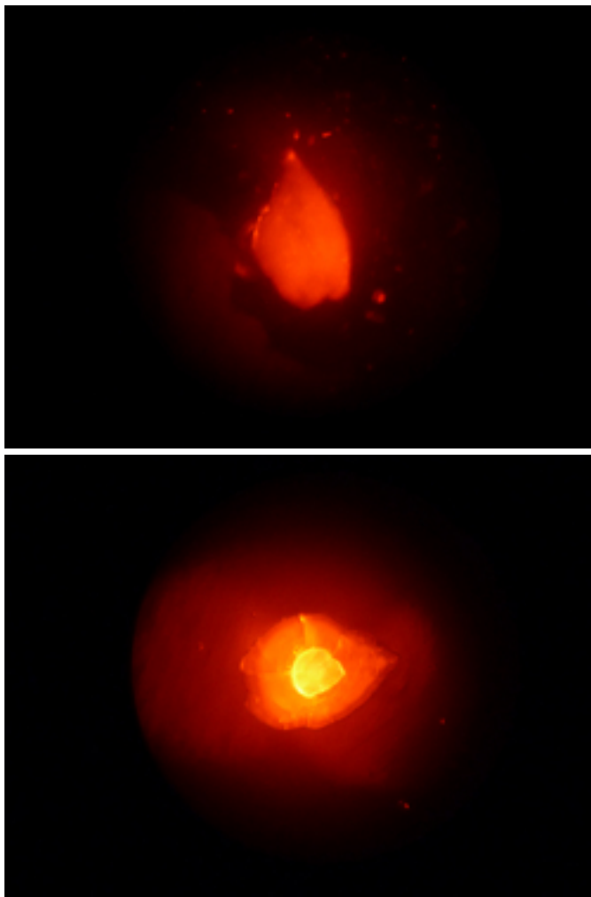
Figure 3 : À gauche, un otolithe non marqué, à droite, un otolithe marqué. Les poissons de repeuplement qui ont absorbé le colorant peuvent être identifiés des années plus tard par simple examen microscopique.
