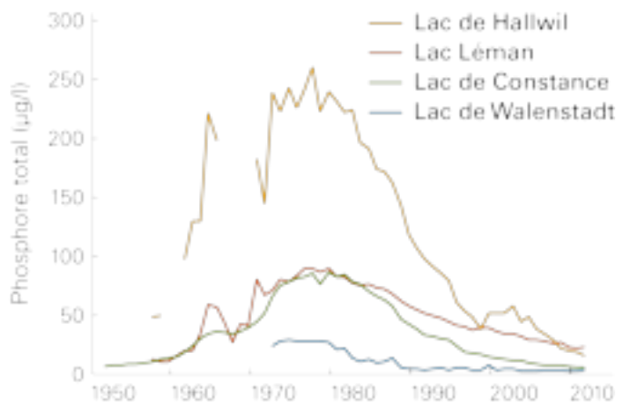
Figure 2 : Évolution des teneurs en phosphore dans 4 lacs suisses de 1950 à 2010. Les apports excessifs de matières nutritives ont des conséquences dramatiques sur les conditions d'oxygénation des profondeurs et peuvent, de ce fait, limiter voire empêcher la reproduction naturelle des salmonidés.
